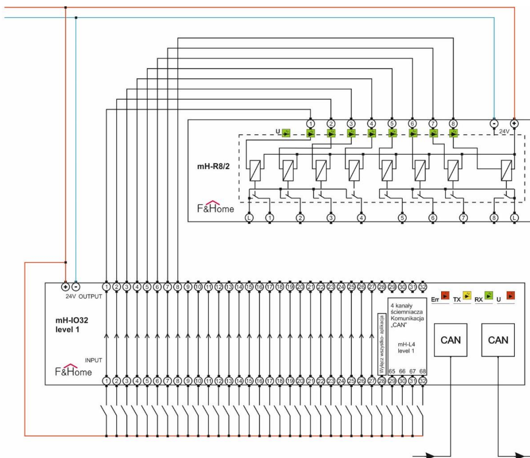
Podłączenie modułu wykonawczego (przełączników – mH-R8x8) do modułu wejść-wyjść.
